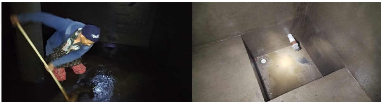
Lavado y desinfección del tanque de distribución, en el Sistema de Agua Potable del Caserío Chuacruz, San José Chacayá, Sololá.
