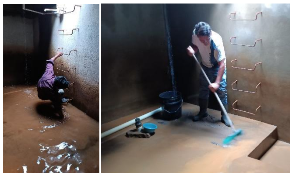
Lavado y desinfección de tanque de distribución, del sistema de agua potable del Caserío San Felipe, San José Chacayá, Sololá.
